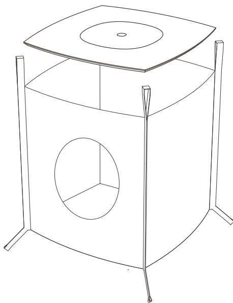
Colación da base Introducila base no interior da saca previamente recortada, de xeito que quede ben rechán
