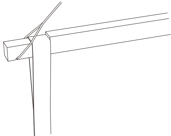
Encontro de esquina entre asa, barrote e corda. Vestila asa da saca ate o final do rebaixe e logo encaixala corda na ranura.
