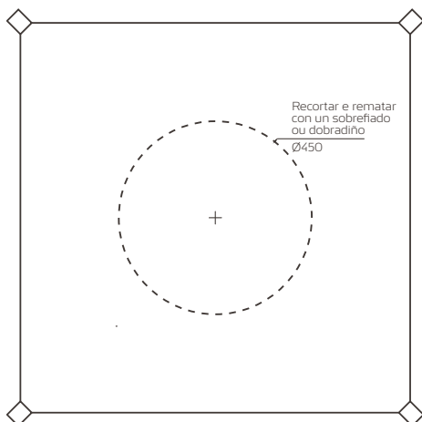
Planta Saca grande de rafia ou Big/Bag 900x900x1000 mm.
