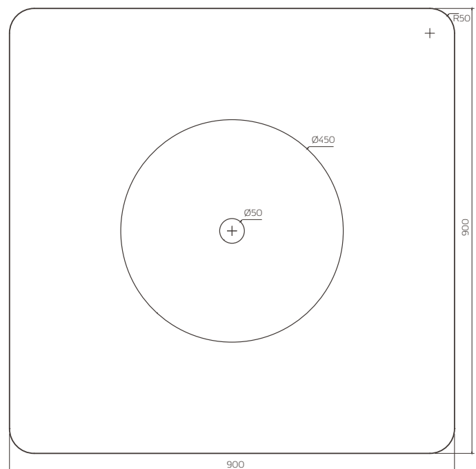
Planta Base interior con tapa de tableiro contrachapado e. 20mm.
